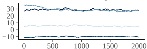
b_lockdown_step4
