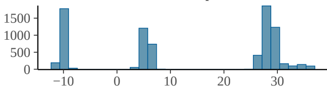
b_lockdown_planB
