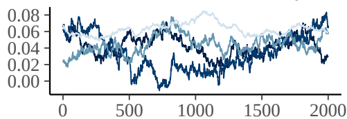
b_scale_carehome_density
