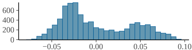
b_scale_prop_urb
