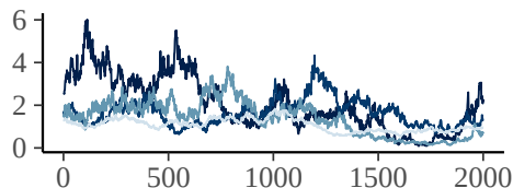
sds_sdate_index_1
