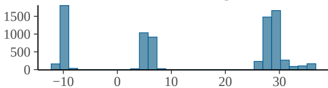
b_lockdown_step3
