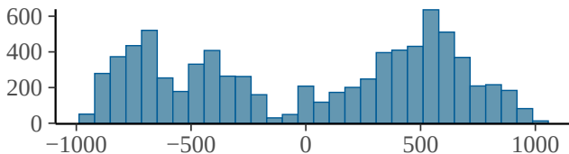
bs_sdate_index_1
