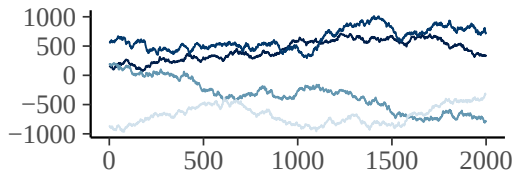
bs_sdate_index_1
