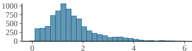
sds_sdate_index_1
