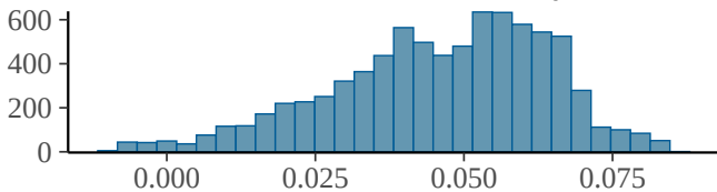
b_scale_carehome_density
