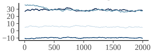
b_lockdown_step3
