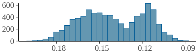
b_scale_BAME
