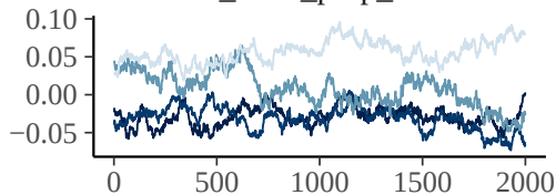
b_scale_prop_urb
