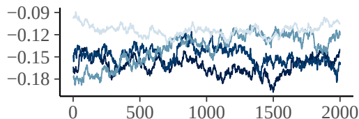
b_scale_BAME
