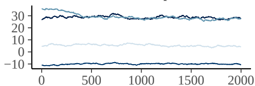
b_lockdown_planB
