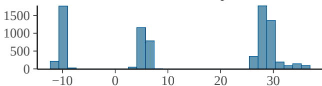
b_lockdown_step4
