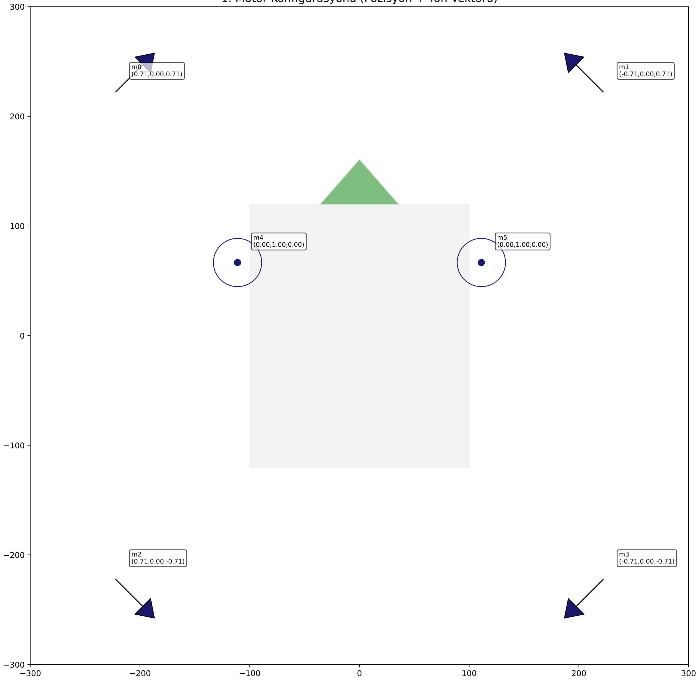
1. Motor Konfigürasyonu (Pozisyon + Yön Vektörü)
