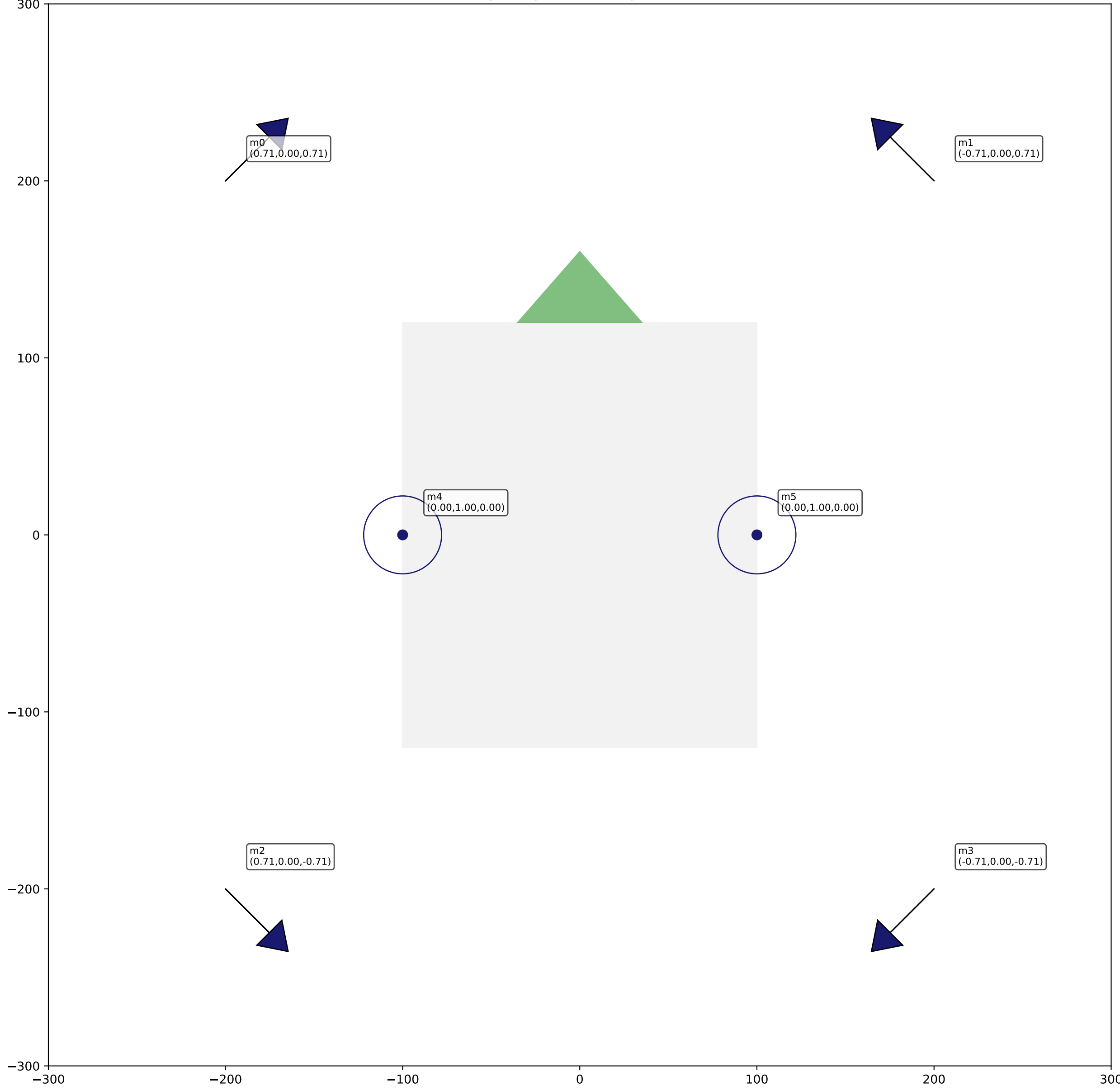
1. Motor Konfigürasyonu (Pozisyon + Yön Vektörü)
