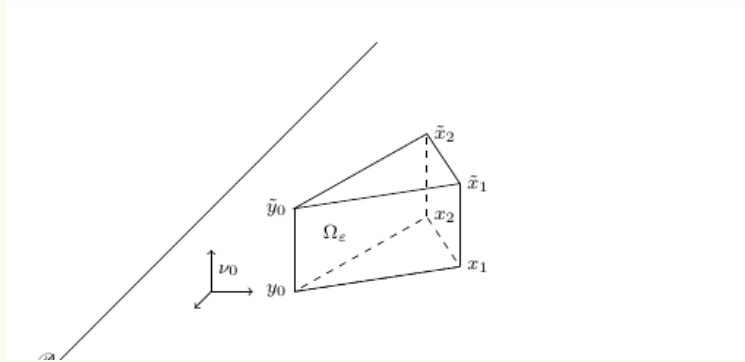
图 1: 棱柱 \Omega_\varepsilon
