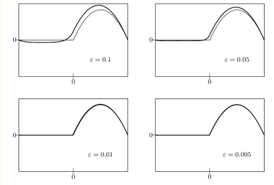
图 VII.3: \varepsilon = 0.1, 0.05, 0.01, 0.005 时精确解 (细线) 与罚解 (粗线) 的整体形状.
