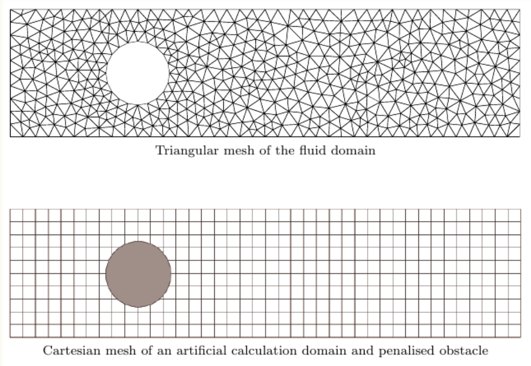
图 VII.2: 计算圆柱绕流的经典方法与罚方法.
