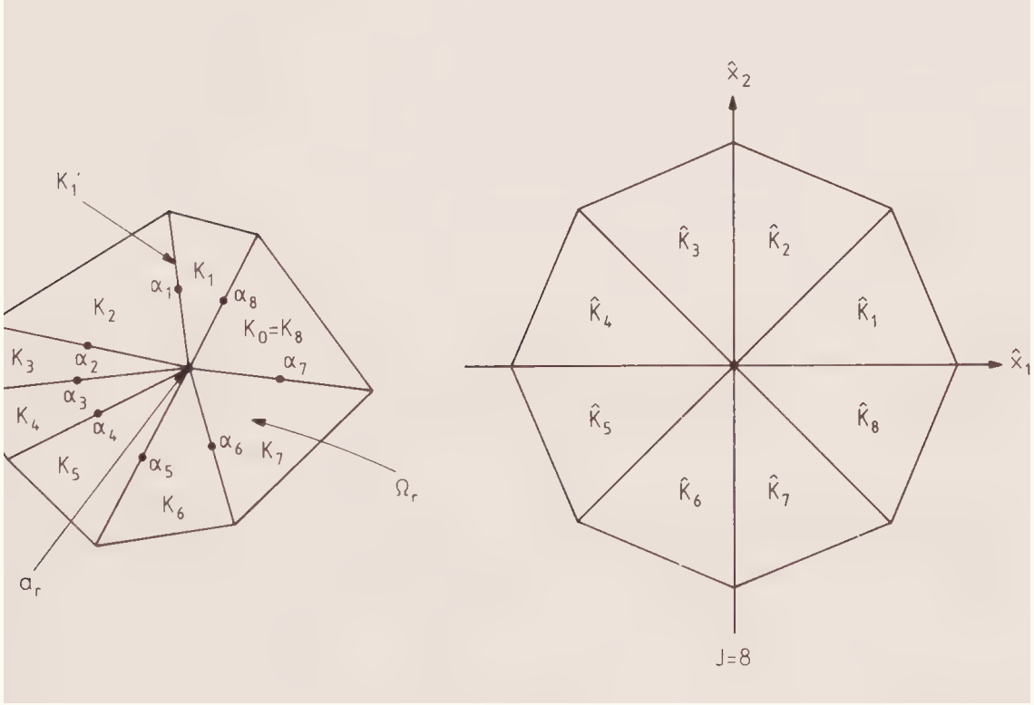
图 18: 一个宏单元及其参考宏单元.
