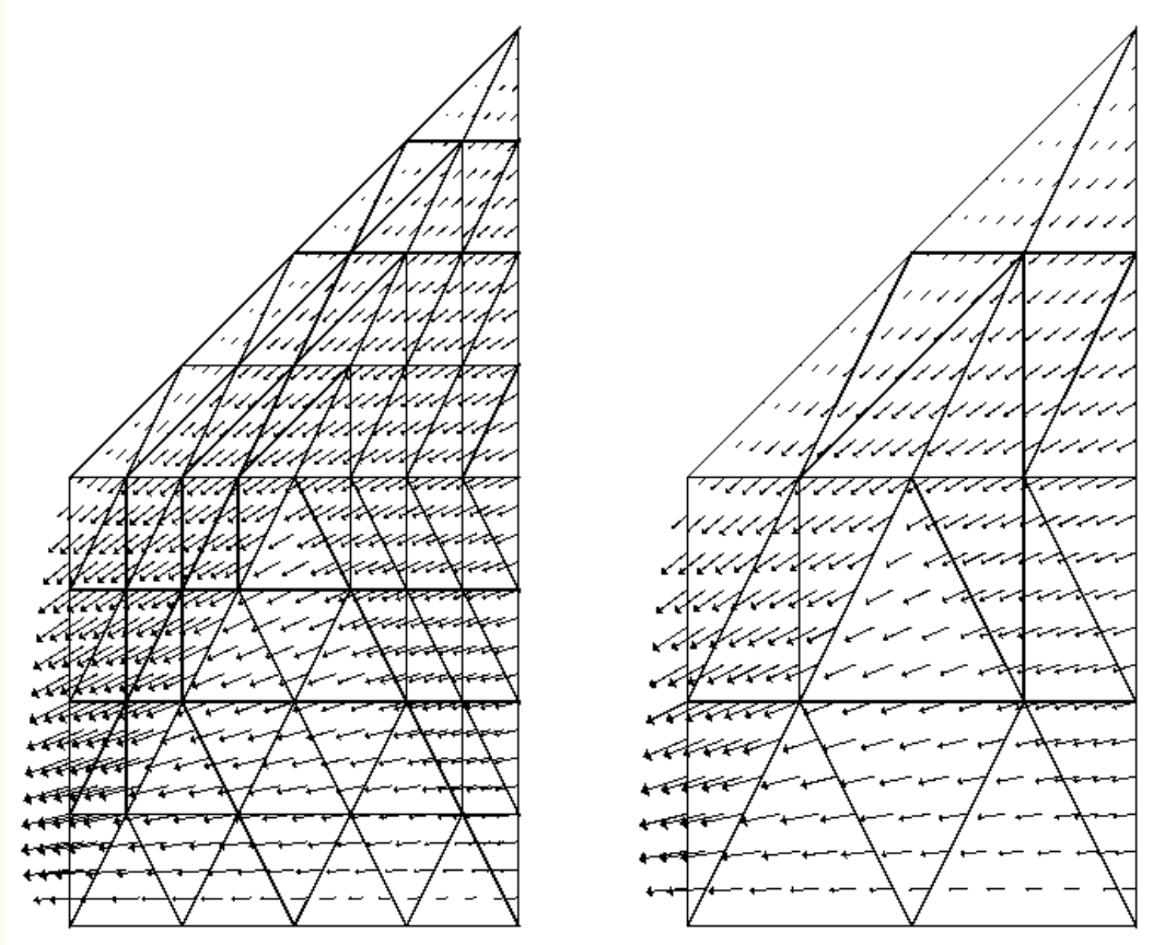
图 13.12: 用四次和六次分片多项式计算的 Jeffrey–Hamel 流.
