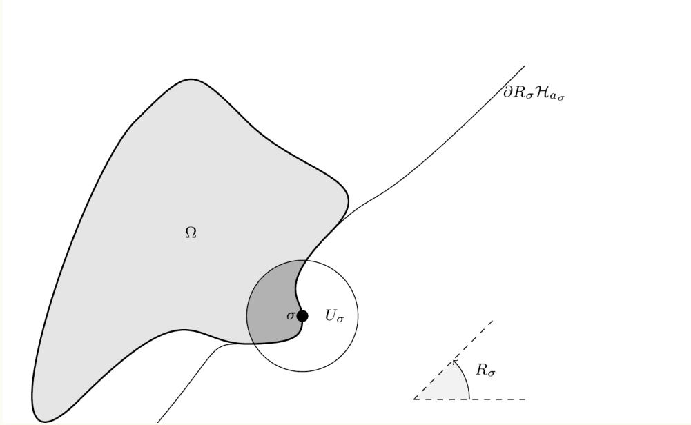
图 III.1: C^{k, \alpha} 区域局部为 C^{k, \alpha} 半空间.
