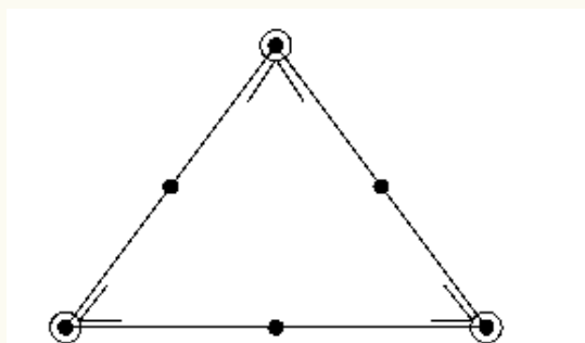
图 3.27: 一个四次有限元
