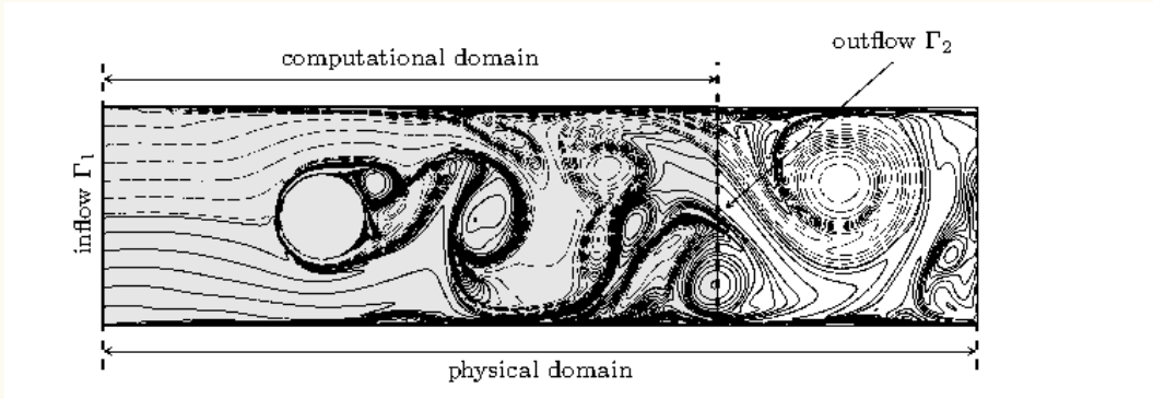
图 VII.1: 为计算目的对物理区域进行截断.
