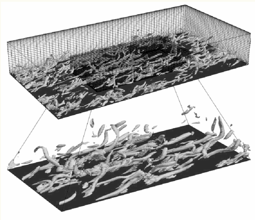
图 16: 无控制通道流的边界层中相干结构的形成.
