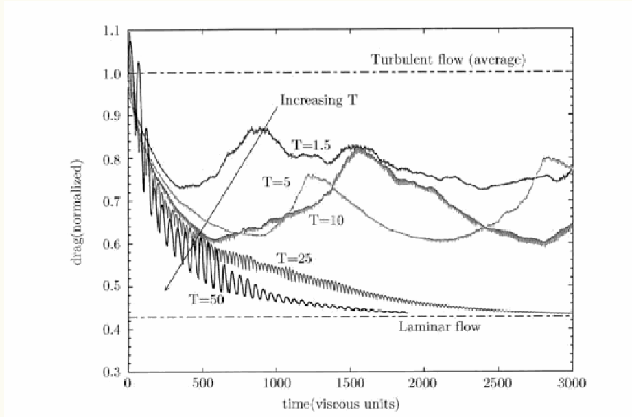
图 17: 受控流中, 不同参数 T 取值对应的阻力随时间演化.
