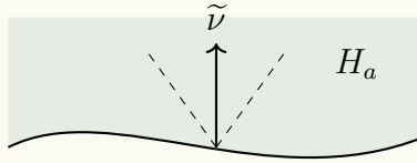
图 III.2: 半空间 H_a 及其内锥.
