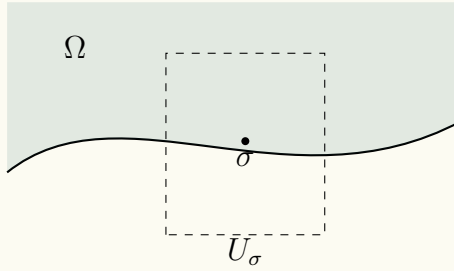
图 III.1: C^{k,\alpha} 区域局部为 C^{k,\alpha} 半空间.
