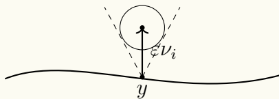
图 III.3: 球 B(y + \varepsilon \nu_i, 2\varepsilon) 包含于锥 C_i .
