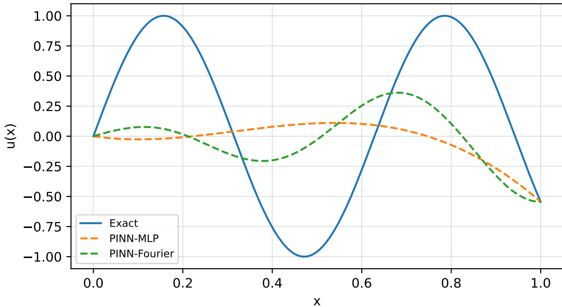
Helmholtz PINN: k=10
