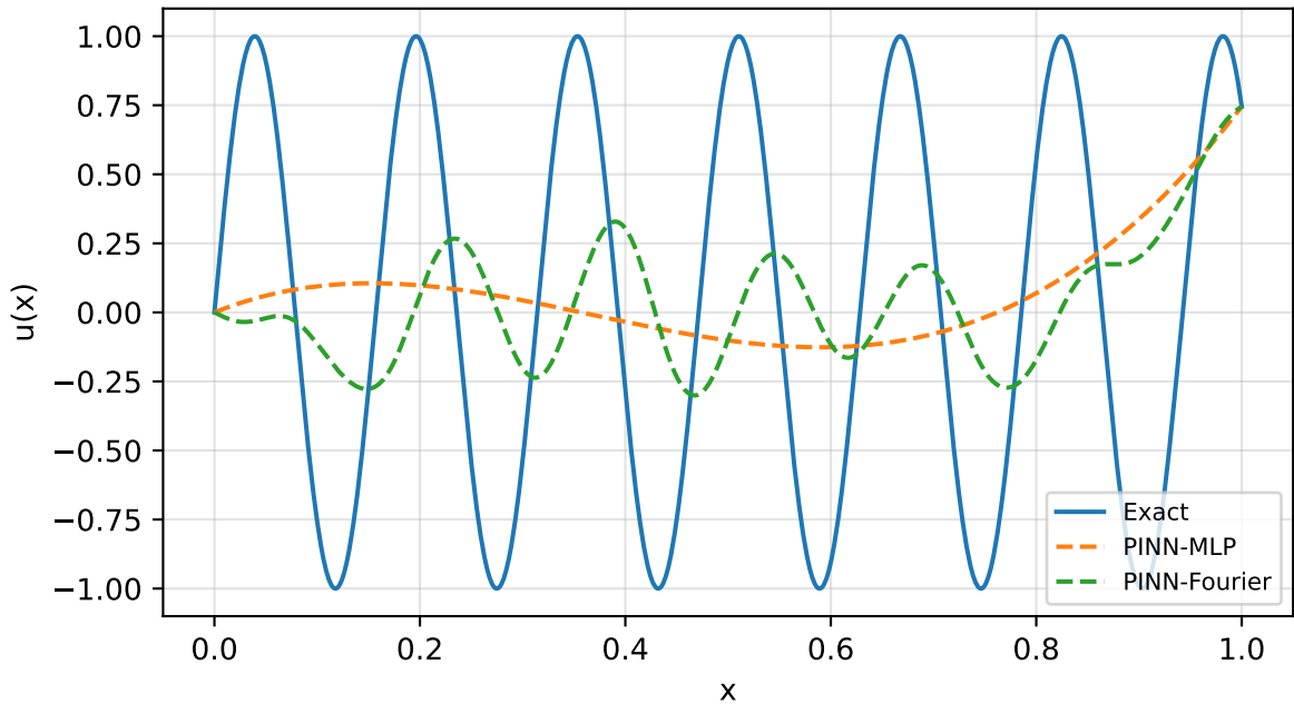
Helmholtz PINN: k=40
