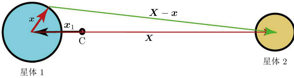
图 1：潮汐问题的示意图
