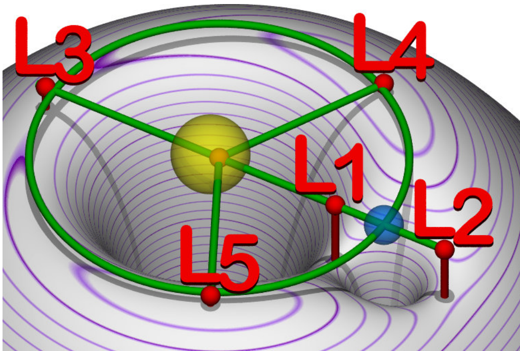
图 3: 日地系统中的五个 Lagrange 点的示意图（比例并不正确）。图中还显示了有效势能 V_{\text{eff}}(\mathbf{x}) 的等高线。需要注意的是，这个图中 x 轴的设定与我们文中是相反的，即如果要与我们文中讨论一致， x 轴的正方向应当向左。
