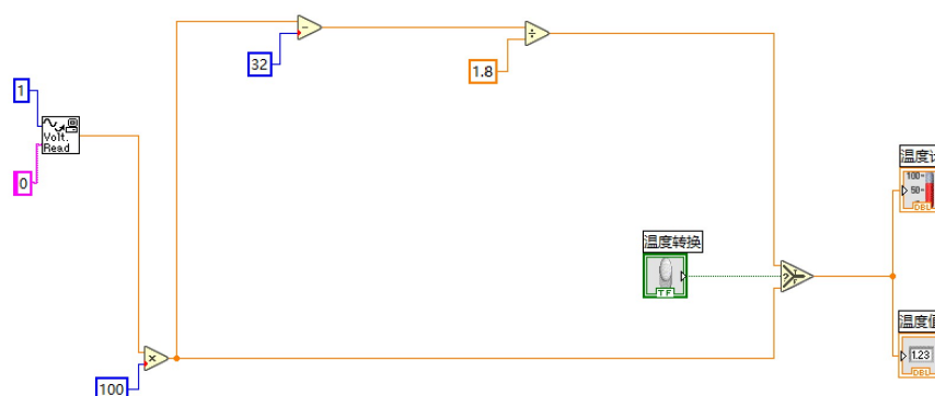
图 1: 模拟温度测量程序的程序框图
