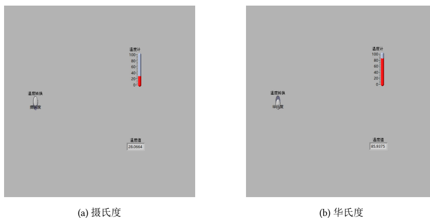
图 2: 程序前面板
