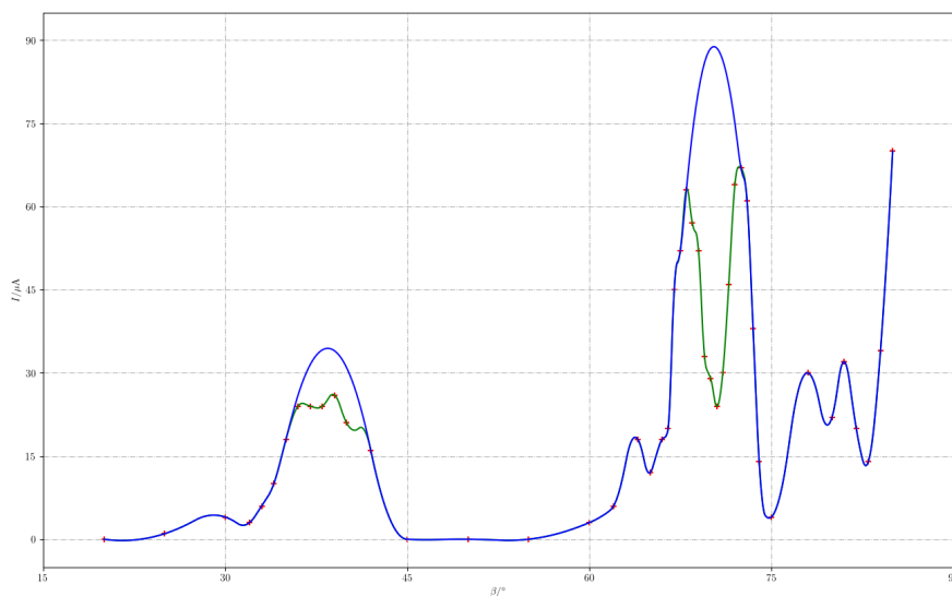
图 1: [100] 晶面的布拉格衍射曲线
