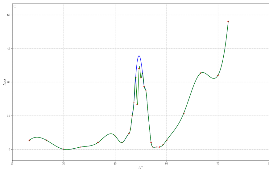
图 2: [110] 晶面的布拉格衍射曲线
