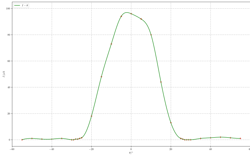
图 3: 微波的单缝衍射
