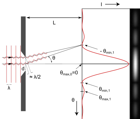
图: 单缝衍射
