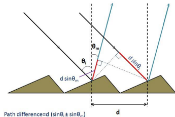
图: 光栅衍射条件
