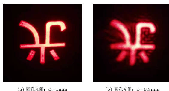
图 6: 高低通滤波实验
