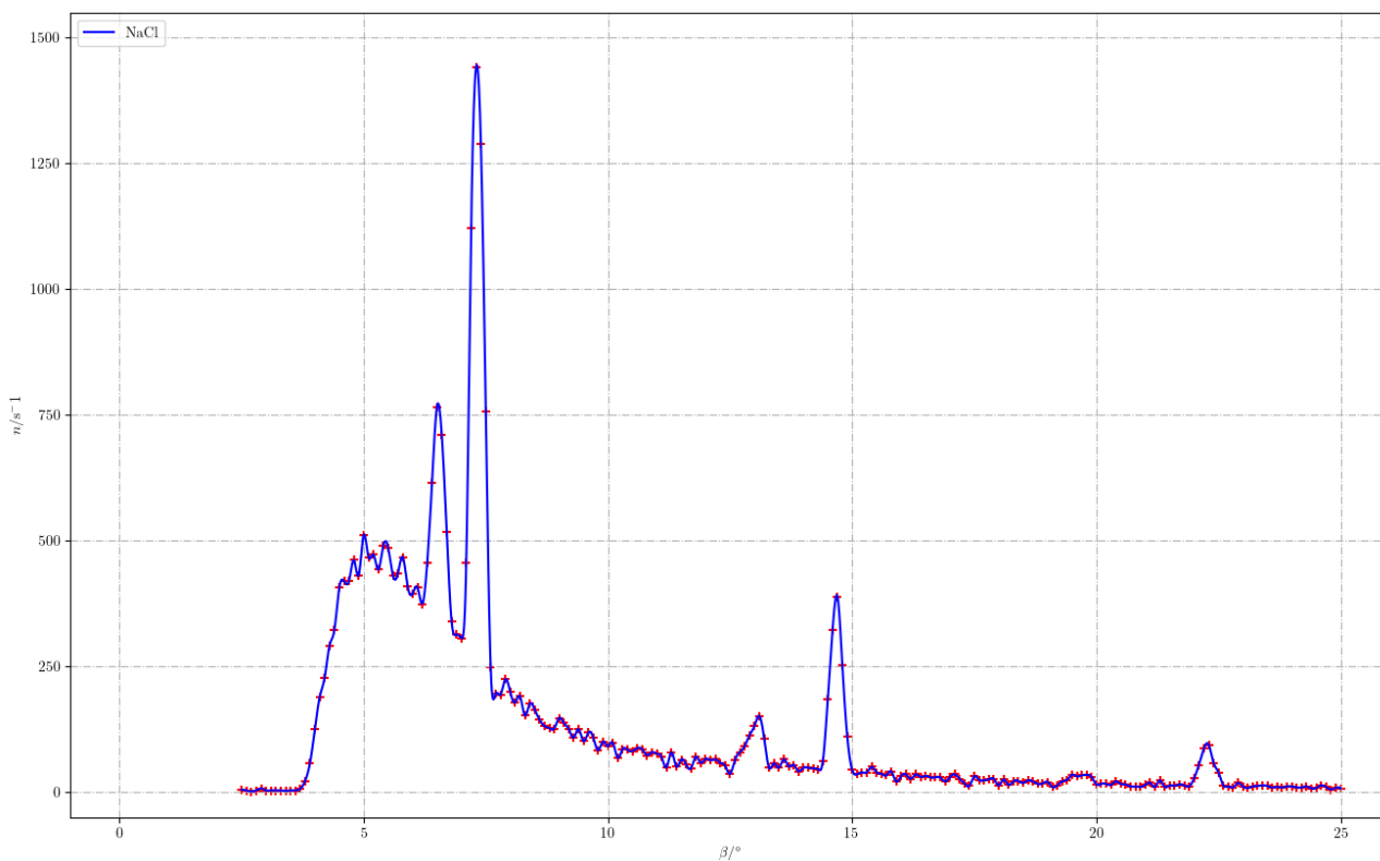
图 1: NaCl 晶体的衍射曲线
