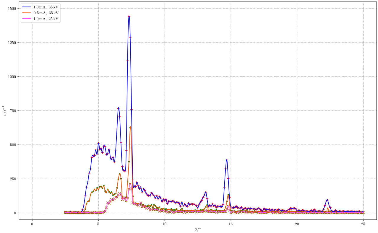
图 3: 三种条件下 NaCl 的衍射曲线
