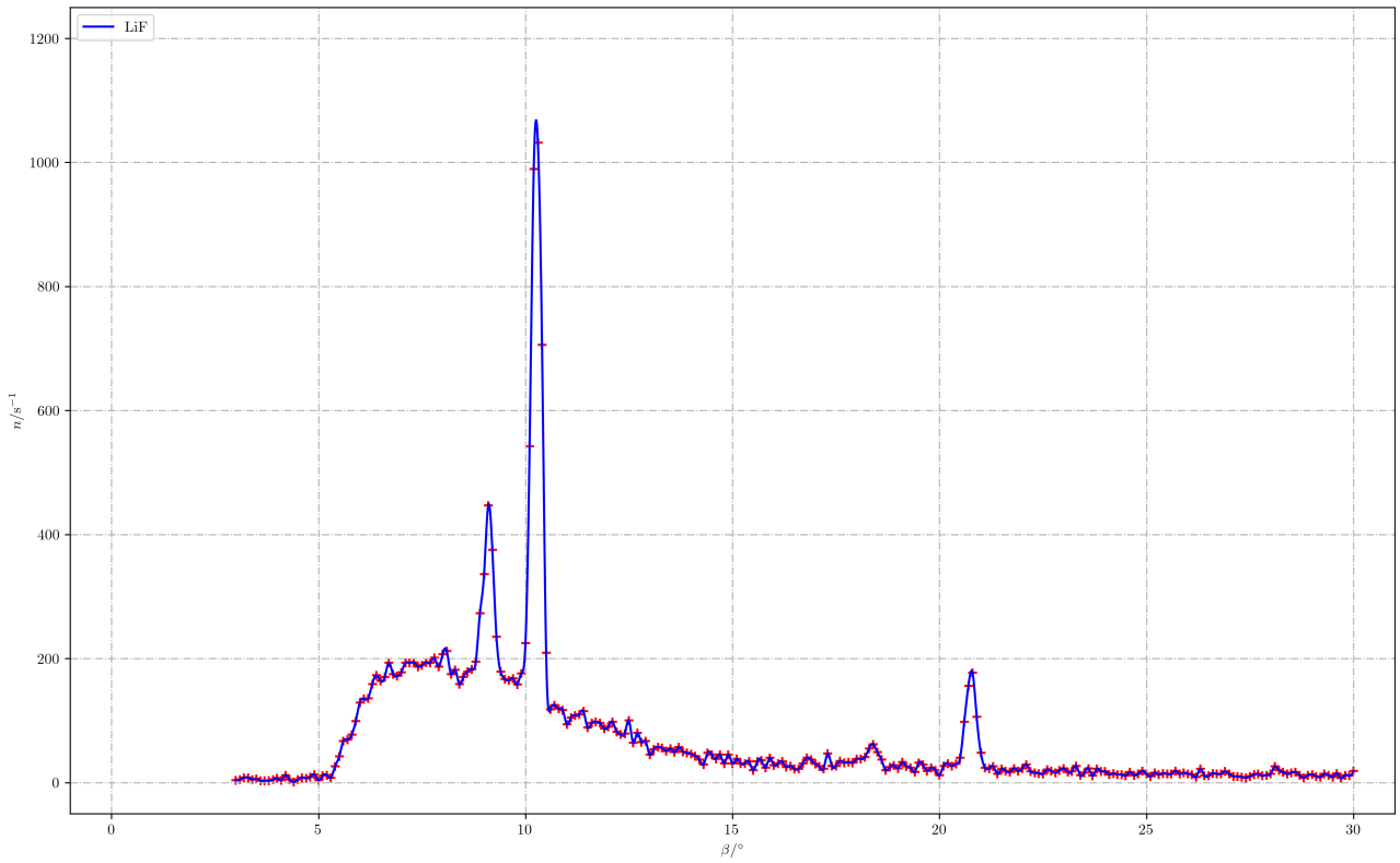
图 2: LiF 晶体的衍射曲线
