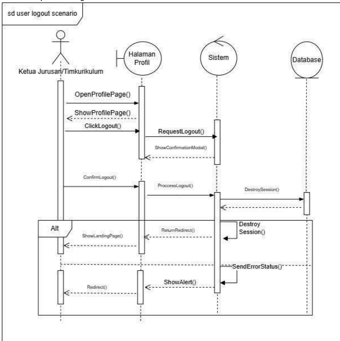
gambar 3.3 sequence diagram keluar dari sistem
