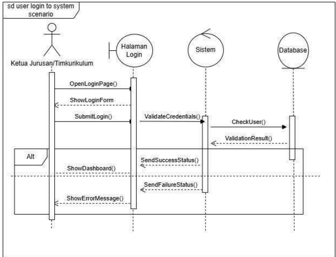
gambar 3.2 sequence diagram masuk ke dalam sistem
