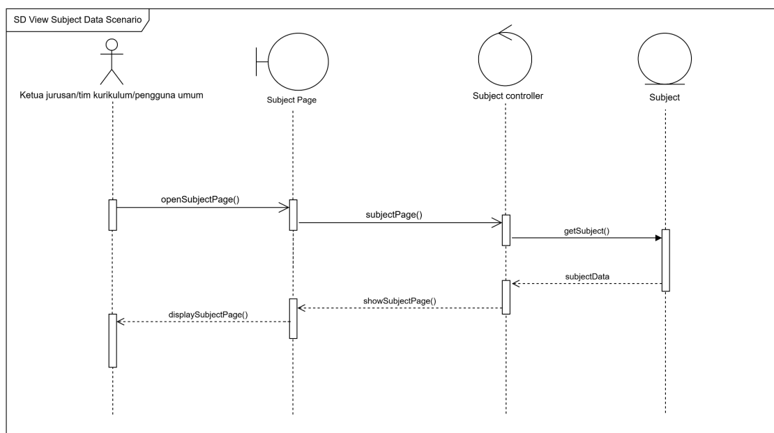
gambar 3.14 sequence diagram melihat data mata kuliah
