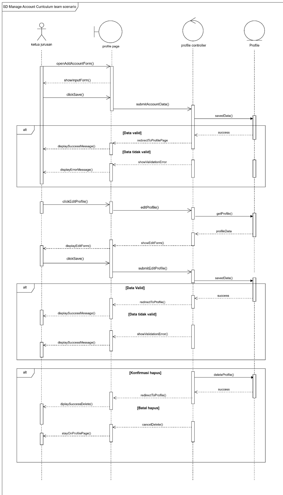
gambar 3.4 sequence diagram mengelola akun tim kurikulum
