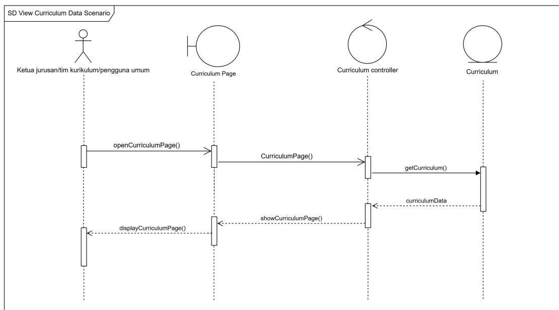
gambar 3.13 sequence diagram melihat data kurikulum
