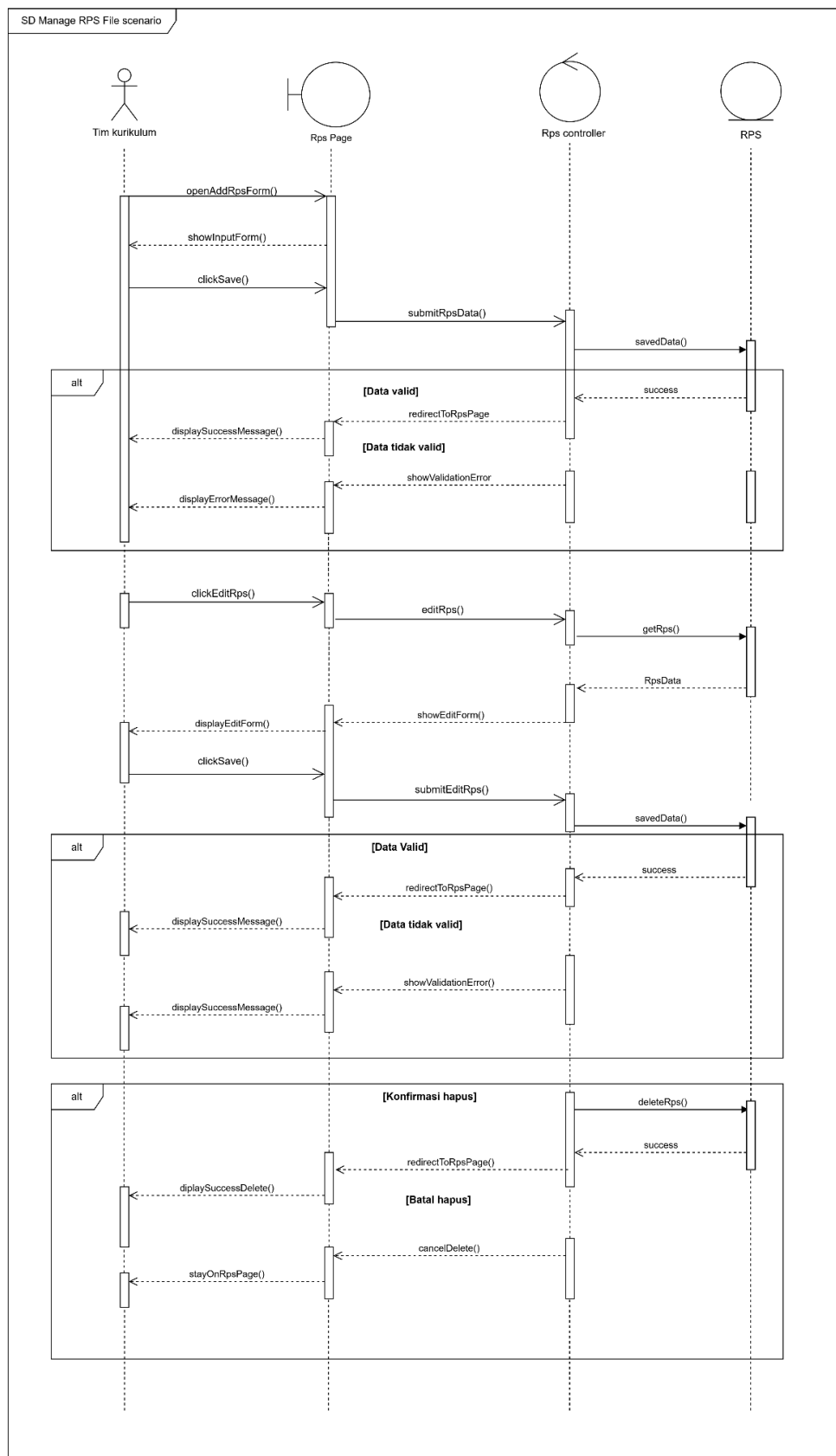
gambar 3.9 sequence diagram mengelola berkas rps
