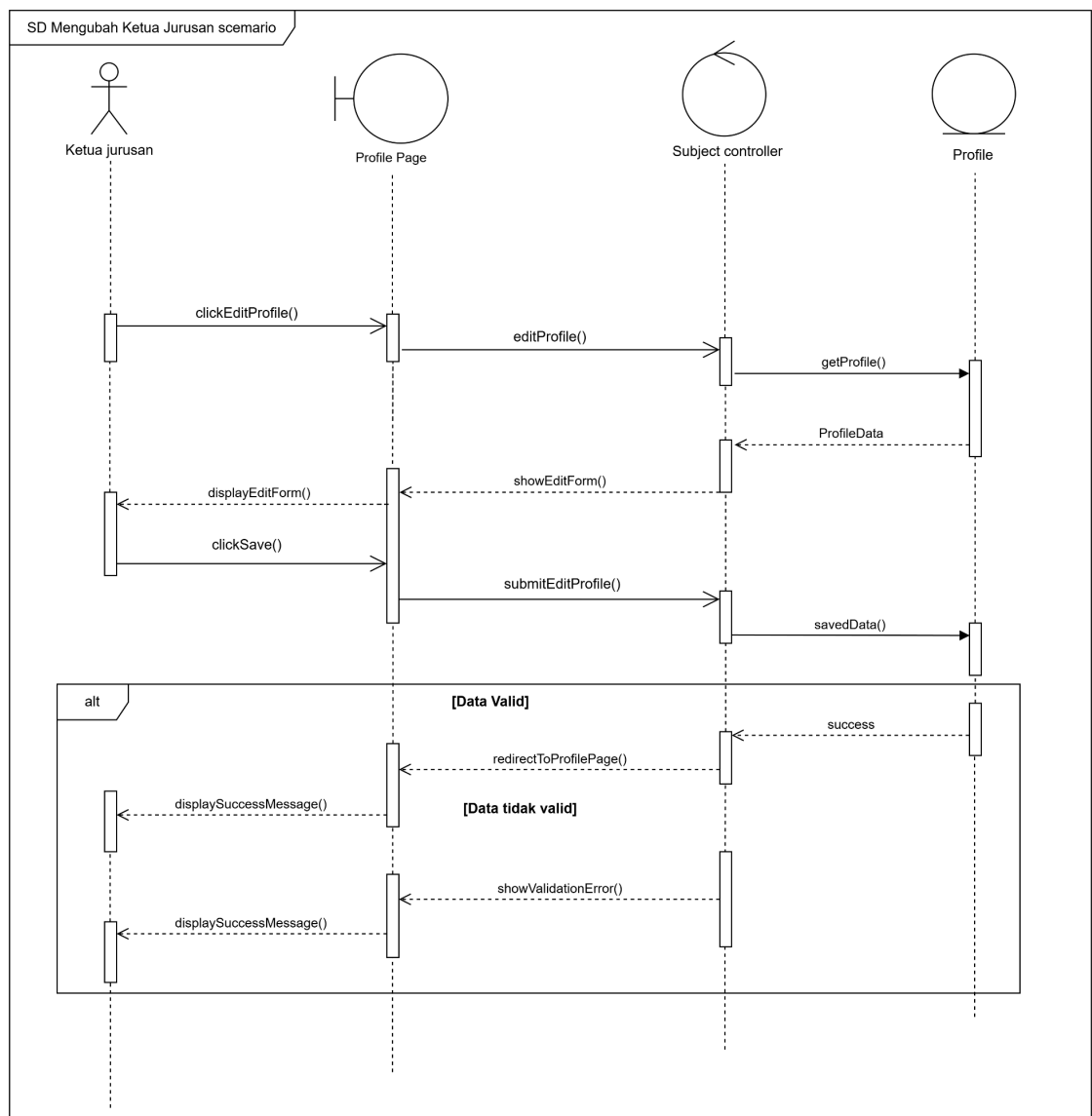
gambar 3.6 sequence diagram mengubah ketua jurusan
