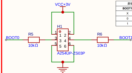
BOOT下载电路
