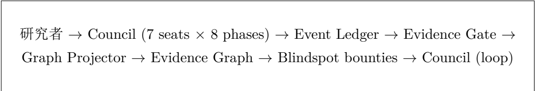
图 1: EpistemoBrain 架构：议会、账本、证据门、投影器与认识论路由形成闭环。过程记忆（左，每席 MemoBrain）与正式证据图（右）物理分离。
