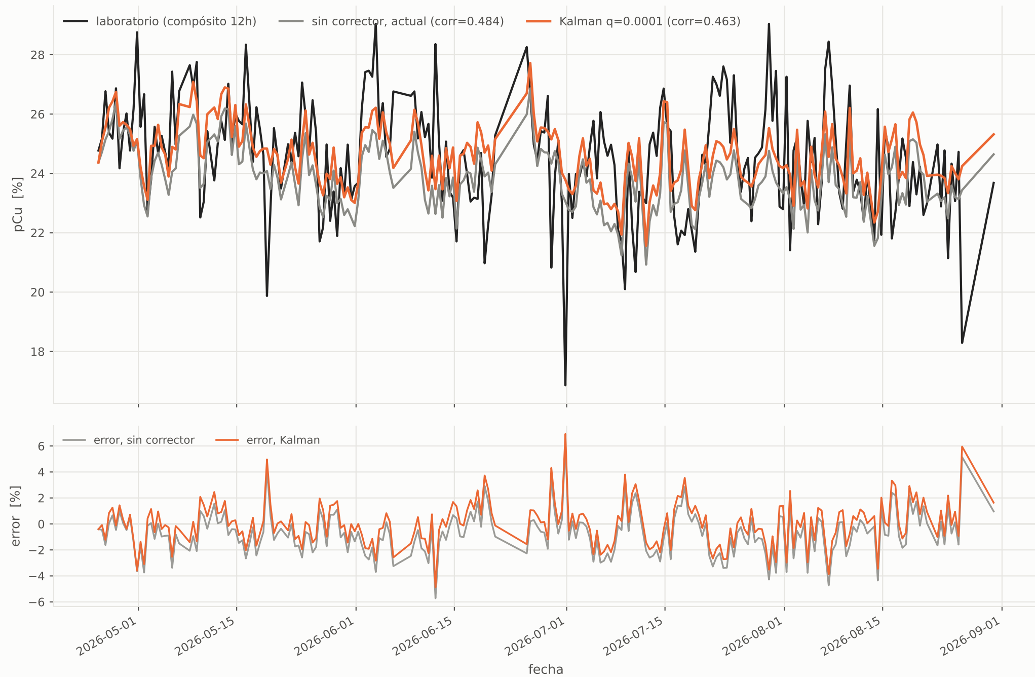
pCu: modelo original sin corrector vs. con corrector Kalman, contra laboratorio
