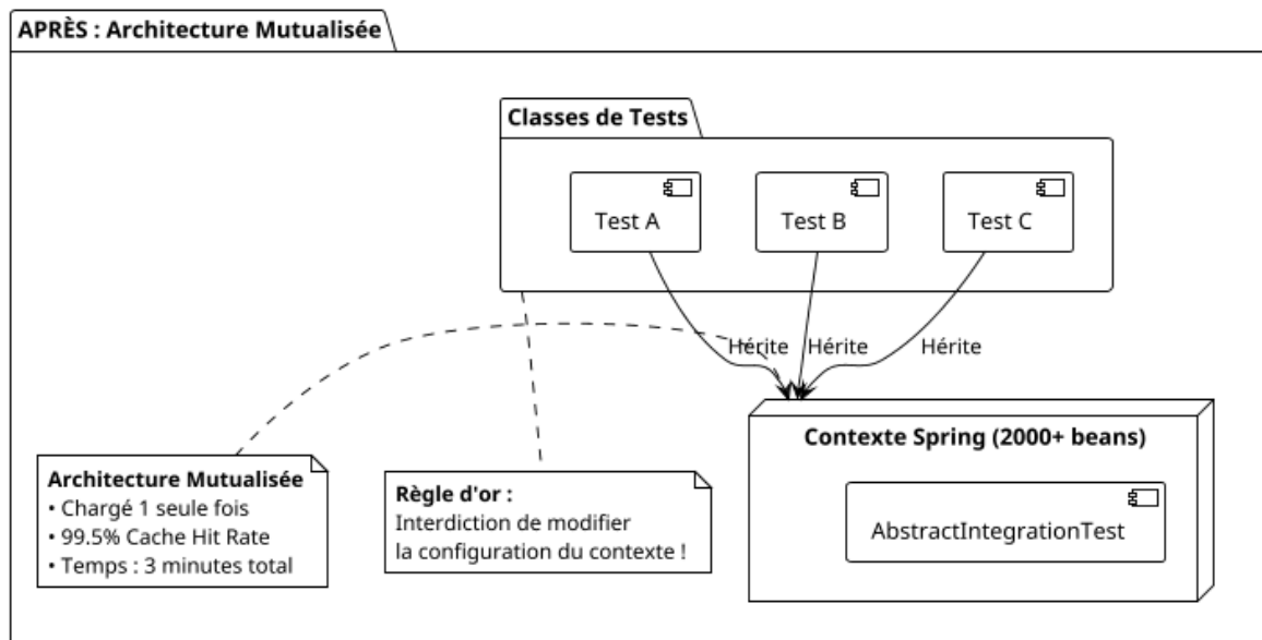
Fig. 2. – Après Optimisation : Mutualisation du contexte Spring Boot pour tous les tests d'intégration.
