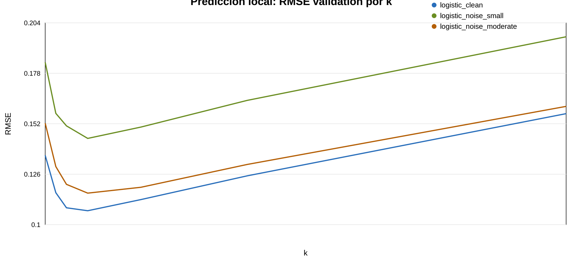
Predicción local: RMSE validation por k
