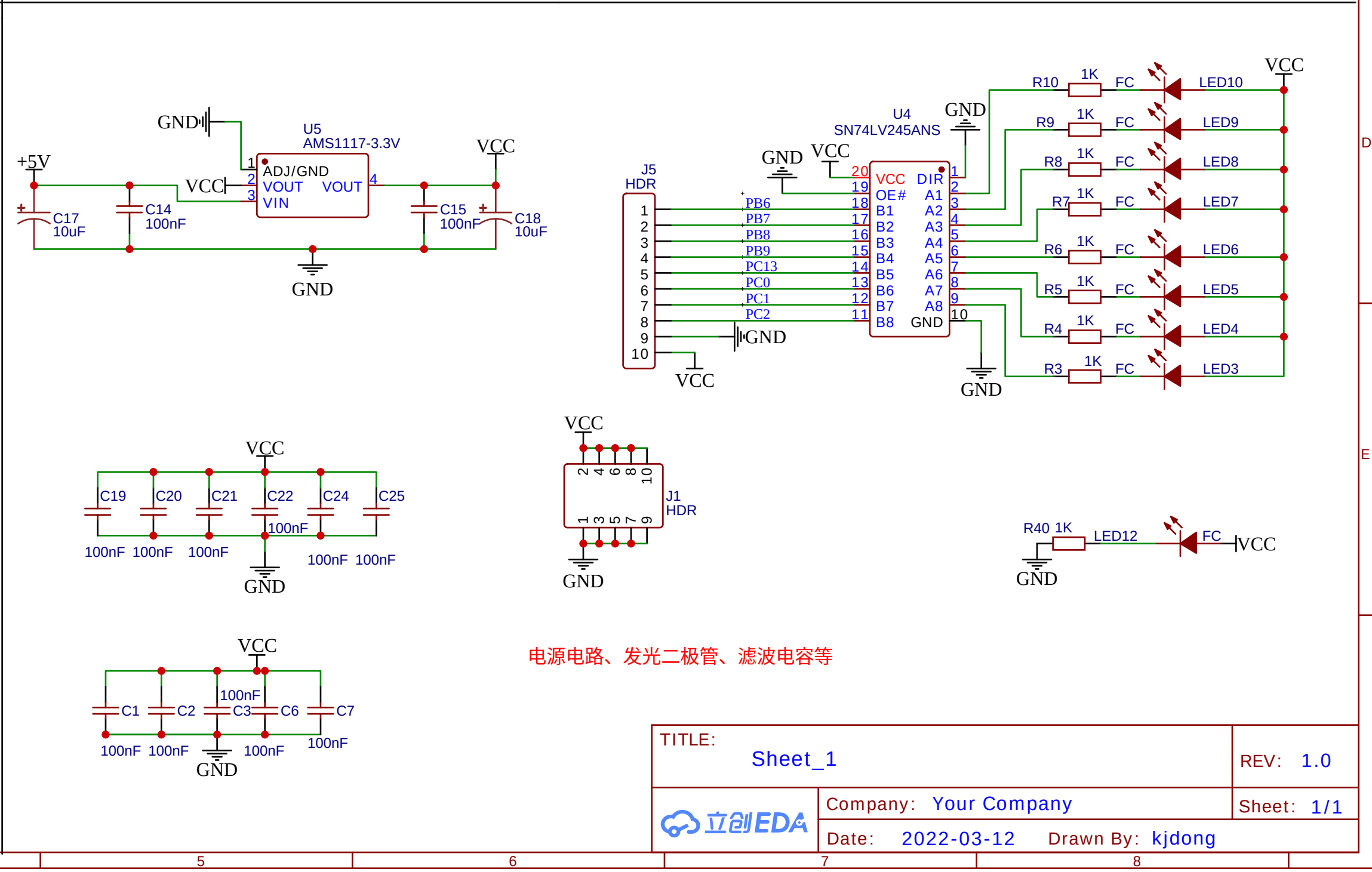
人机对话模块
