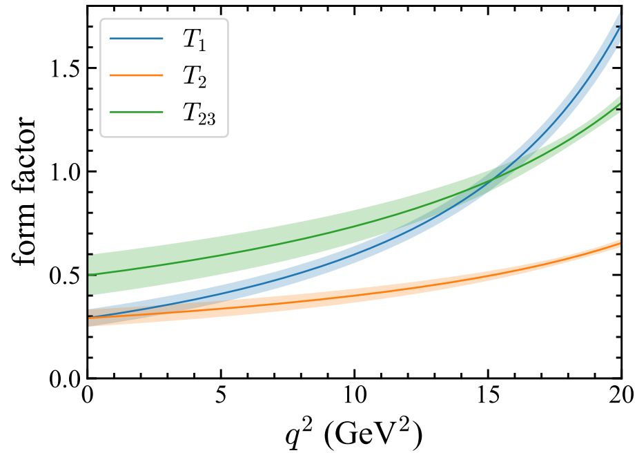
B \rightarrow K^*
