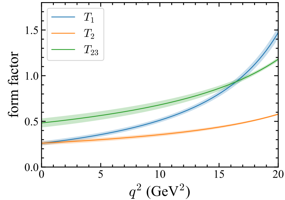
B_s \rightarrow K^*
