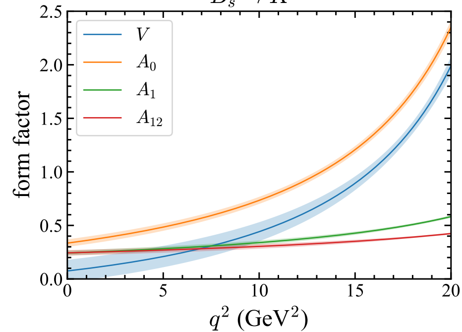
B_s \rightarrow K^*
