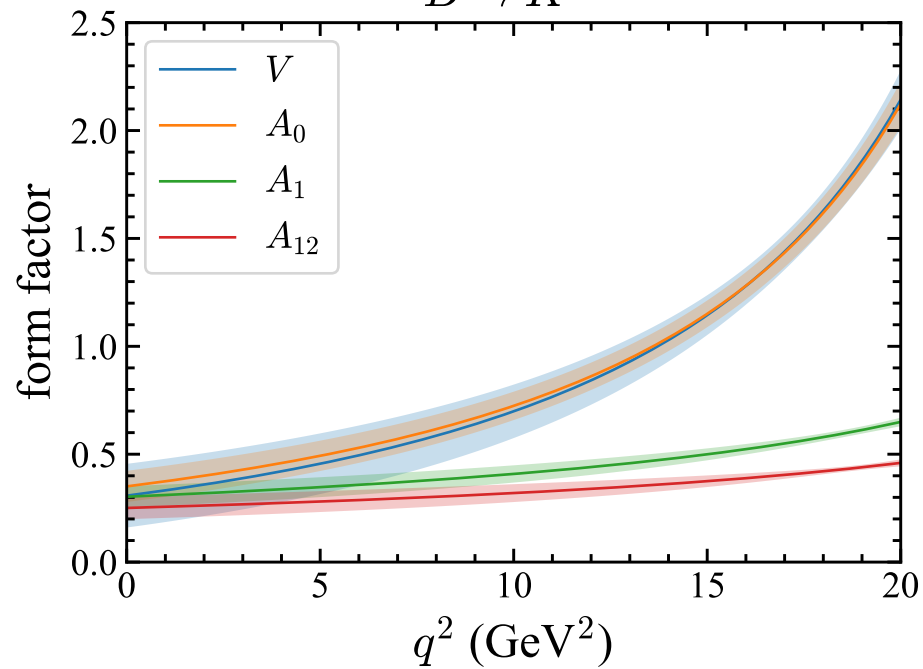
B \rightarrow K^*
