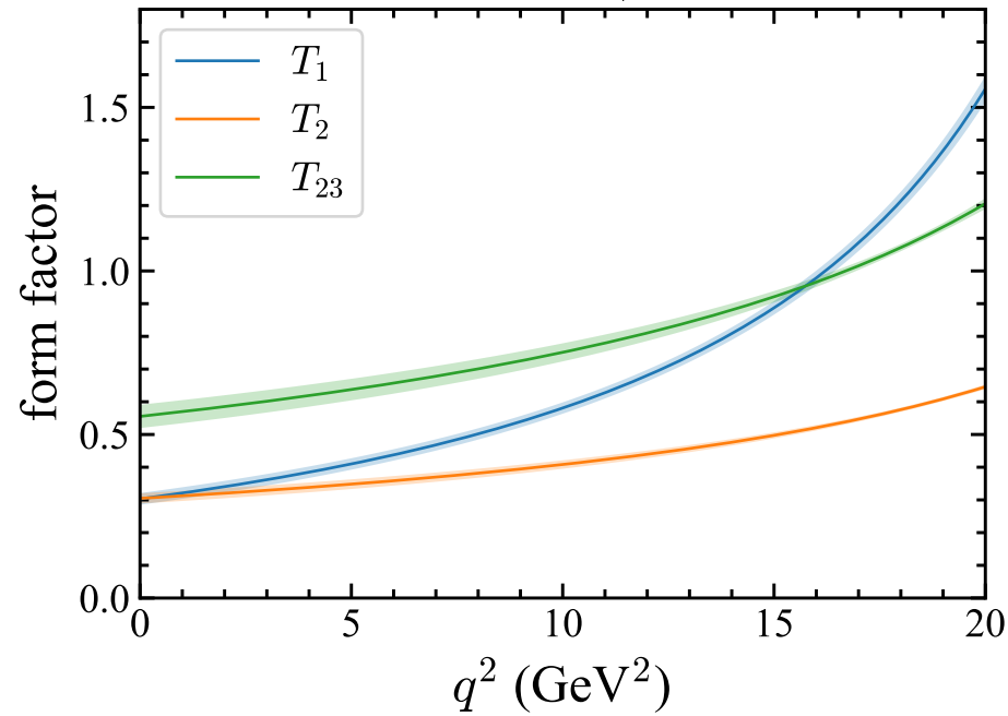
B_s \rightarrow \phi
