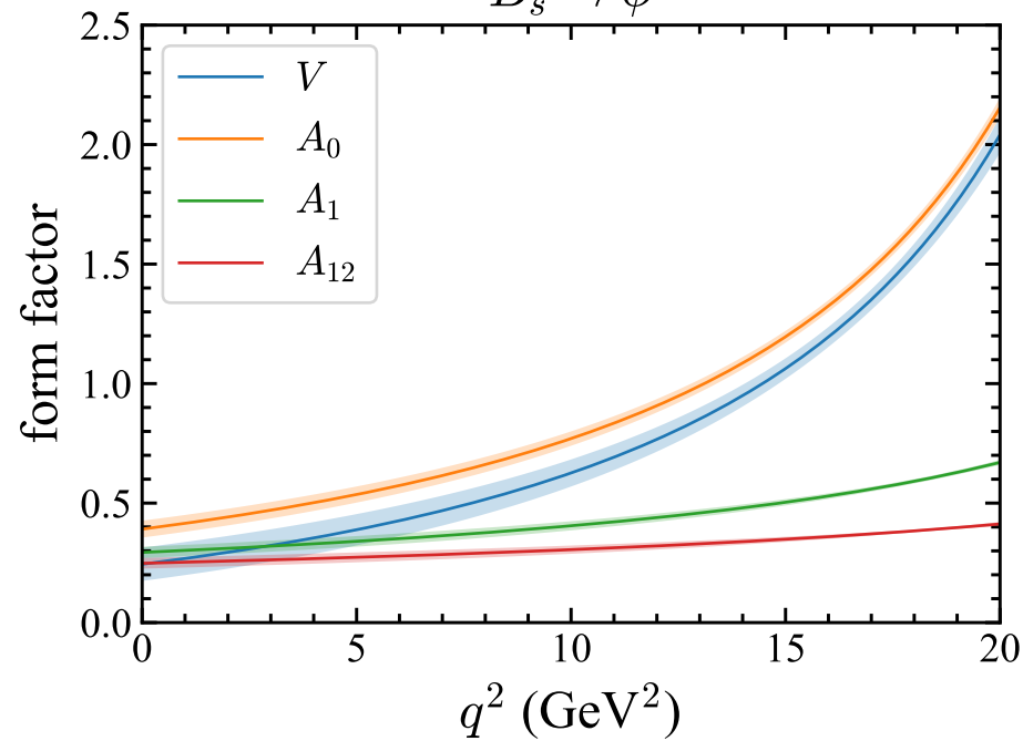
B_s \rightarrow \phi
