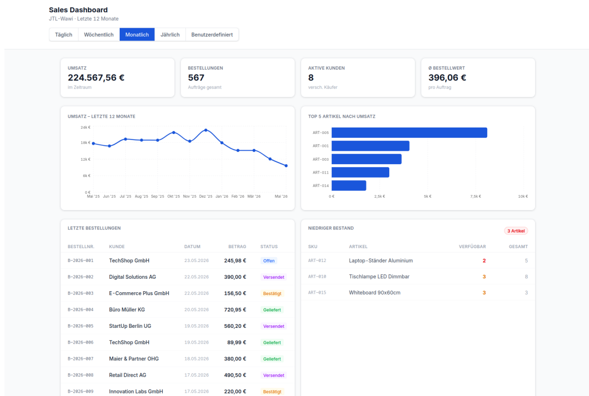
Abbildung 6: Screenshot des fertigen ERP-Dashboards
