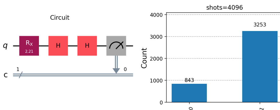
Рис. 21. Квантовая схема к заданию №12
