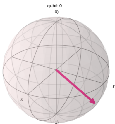
State 1.6.6.png: Bloch
