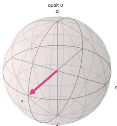
State 1.6.3.png: Bloch
