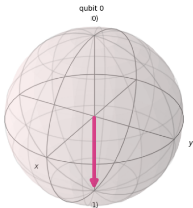
State 1.6.2.png: Bloch
