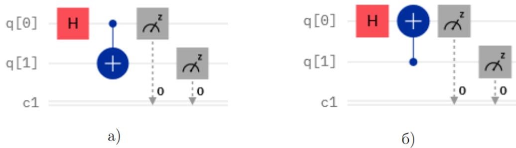
Рис. 17. Квантовые схемы для задания 4
