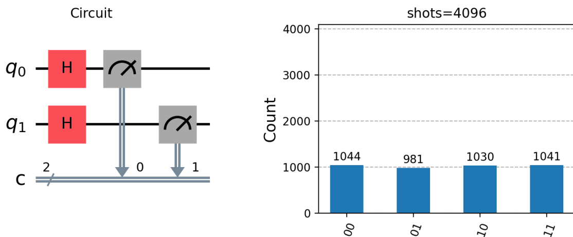
Рис. 23. Квантовые схемы для задания №14
