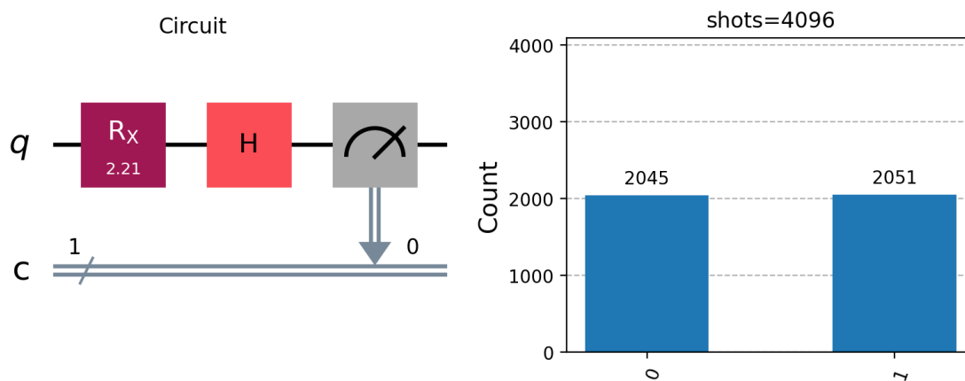
Рис. 20. Квантовая схема к заданию №11
