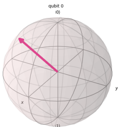
State 1.6.5.png: Bloch
