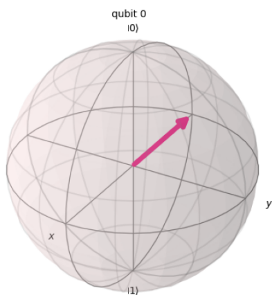
State 1.6.4.png: Bloch
