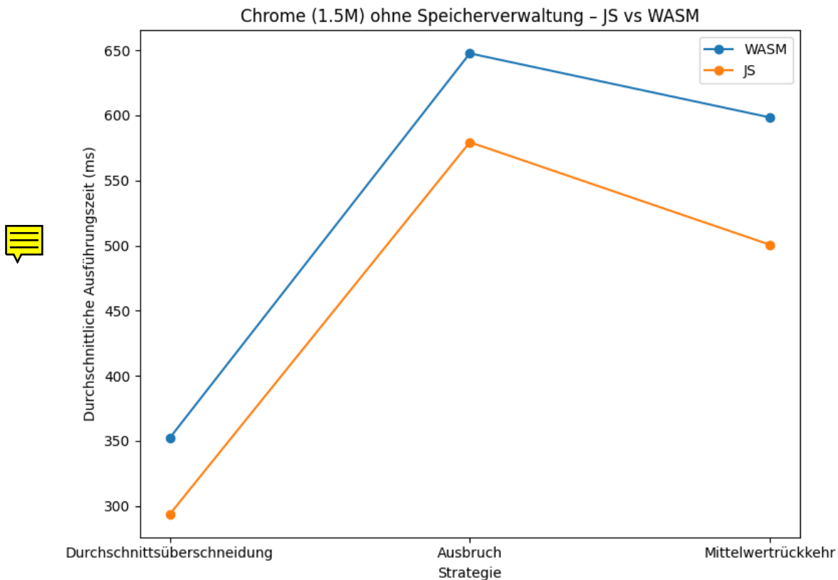
Abbildung 5.9: Durchschnittliche Ausführungszeiten der Strategien ohne Speicherverwaltung in Chrome mit 1,5 Millionen Datenpunkten
