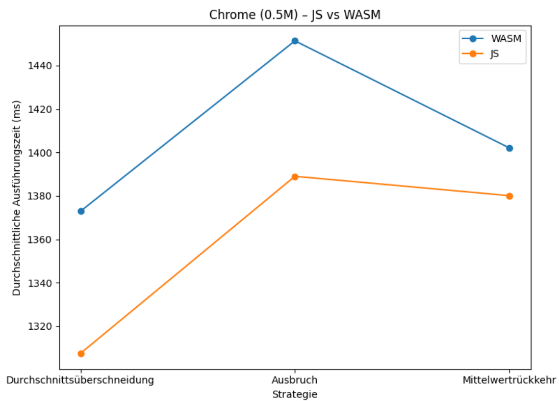
Abbildung 5.3: Durchschnittliche Ausführungszeiten der Strategien in Chrome
