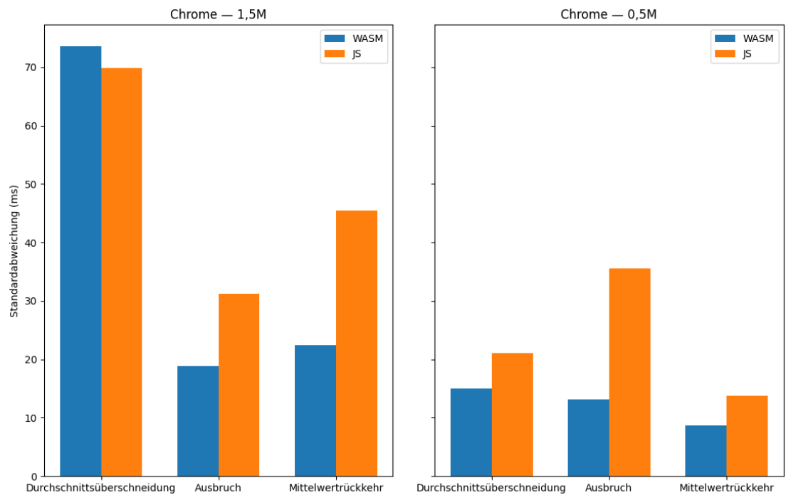
Abbildung 5.5: Standardabweichung der Strategien in Chrome
