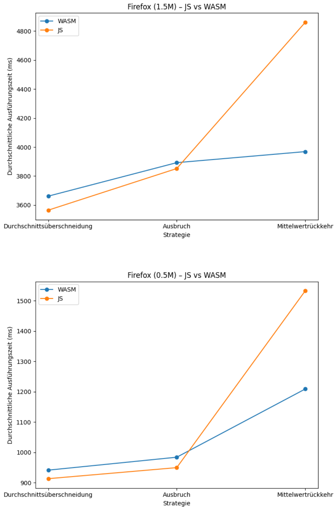
Abbildung 5.2: Durchschnittliche Ausführungszeiten der Strategien in Firefox
