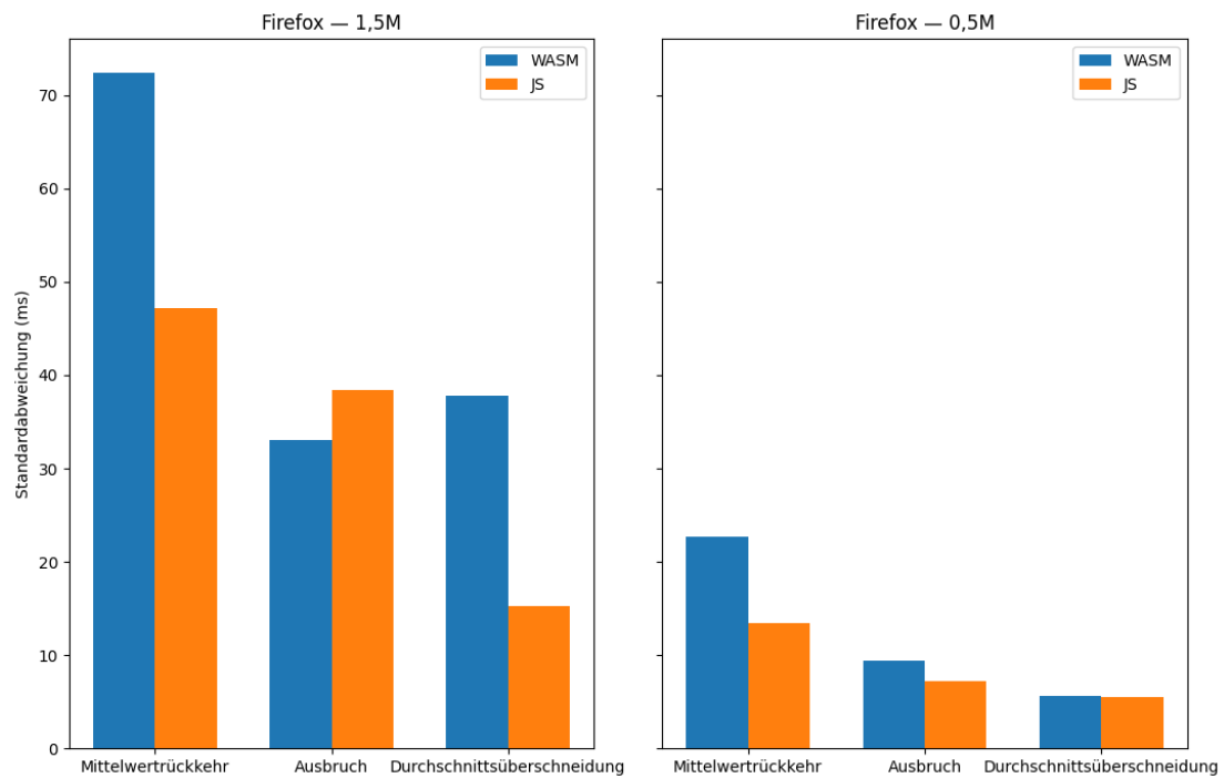
Abbildung 5.4: Standardabweichung der Strategien in Firefox
