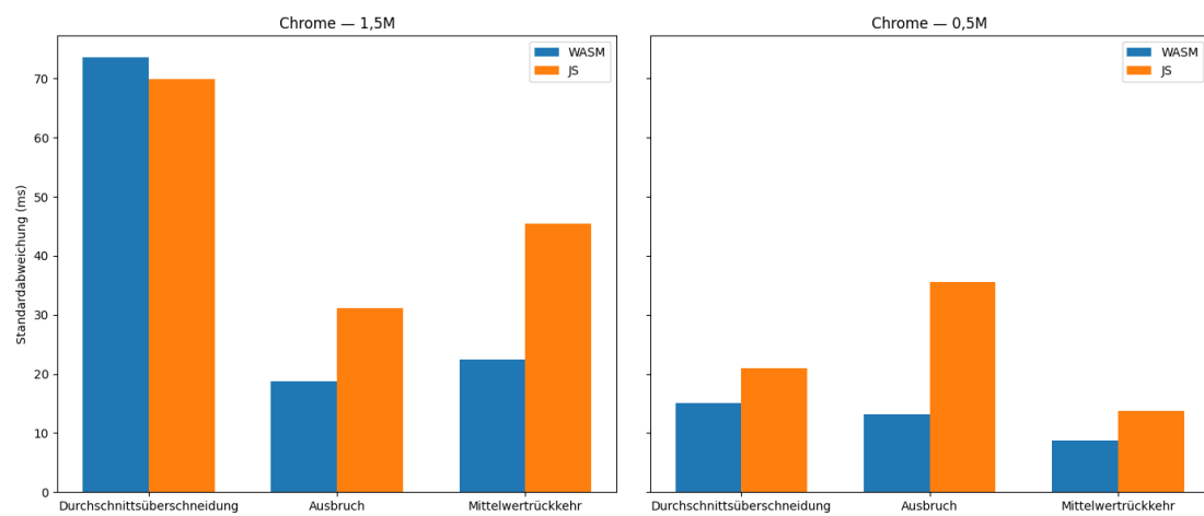
Abbildung 5.5: Standardabweichung der Strategien in Chrome
