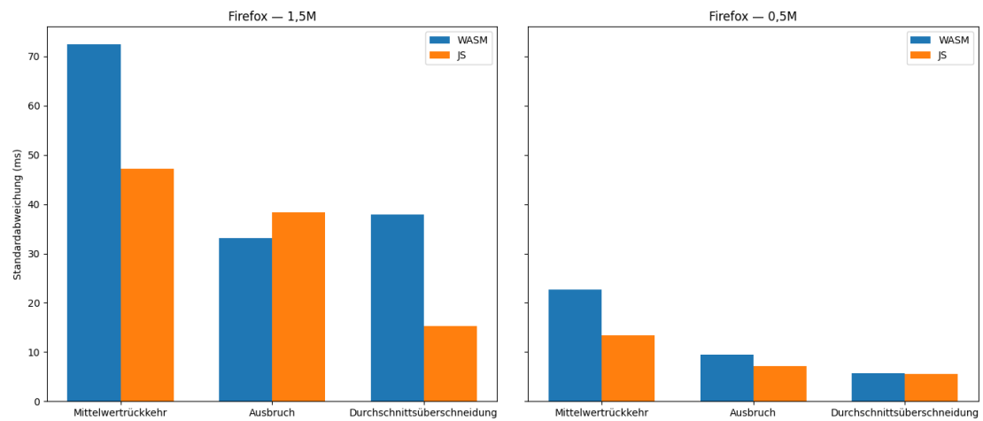
Abbildung 5.4: Standardabweichung der Strategien in Firefox
