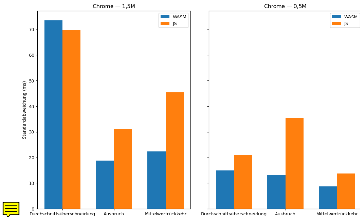
Abbildung 5.7: Standardabweichung der Strategien in Chrome
