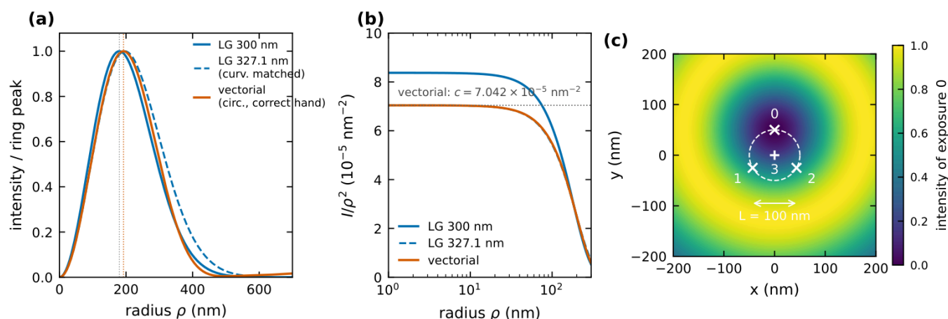
Figura 1. Modelo del trabajo. Perfil radial de la dona LG (fwhm = 300 nm), de la LG igualada por curvatura y de la dona vectorial (a). Curvatura cerca del cero, I/\rho^2 (b). Patrón TCP: 3 donas en un círculo de diámetro L = 100 nm más una en el centro; el mapa muestra la intensidad de una exposición (c). scripts/fig_1_schematic.py [src:fig1]
