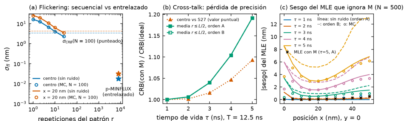
Figura 1. Temporización de p-MINFLUX ( L = 100 , fwhm = 300, T = 12.5 ns). Error por parpadeo: MINFLUX secuencial frente a entrelazado (estrellas) (a). Pérdida de precisión por el cruce entre ventanas con M en el modelo (b). Sesgo del MLE que ignora M ( N = 500 ); las \times corresponden al MLE con M (c). scripts/fig_9_pminflux_timing.py [src:fig9]
