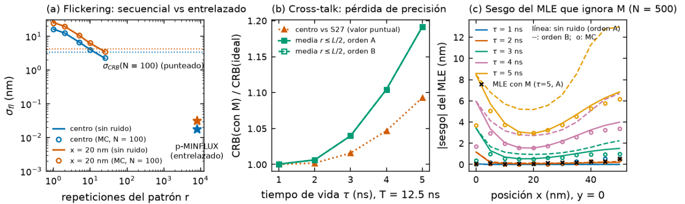
Figura 3. Temporización de p-MINFLUX ( L = 100 nm, fwhm = 300 nm). Error por parpadeo \sigma_{fl} frente al número de repeticiones del patrón en MINFLUX secuencial (líneas y círculos) y con entrelazado a 20 MHz (estrellas) (a). Pérdida de precisión por el cruce entre ventanas cuando M está en el modelo (b). Sesgo del MLE que ignora M , con N = 500 ; las \times negras corresponden al MLE que incluye M (c). Script: scripts/fig_9_pminflux_timing.py ; datos: informe/data/pminflux_timing.json . [src:fig9]
