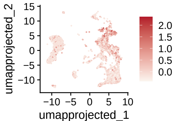
GATA2_EMILIN2_score1
