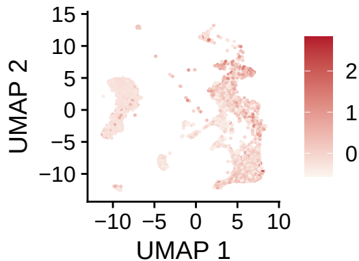
GATA2_EMILIN2_score1
