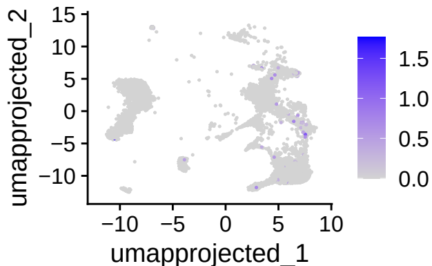
SLC24A3
