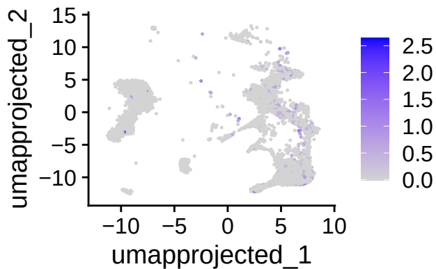
SLC24A3
