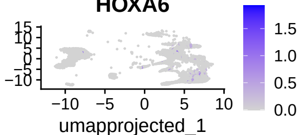
HOXA6
