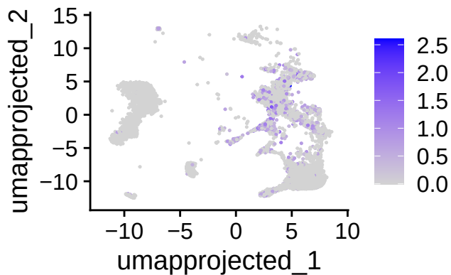
LRP6
