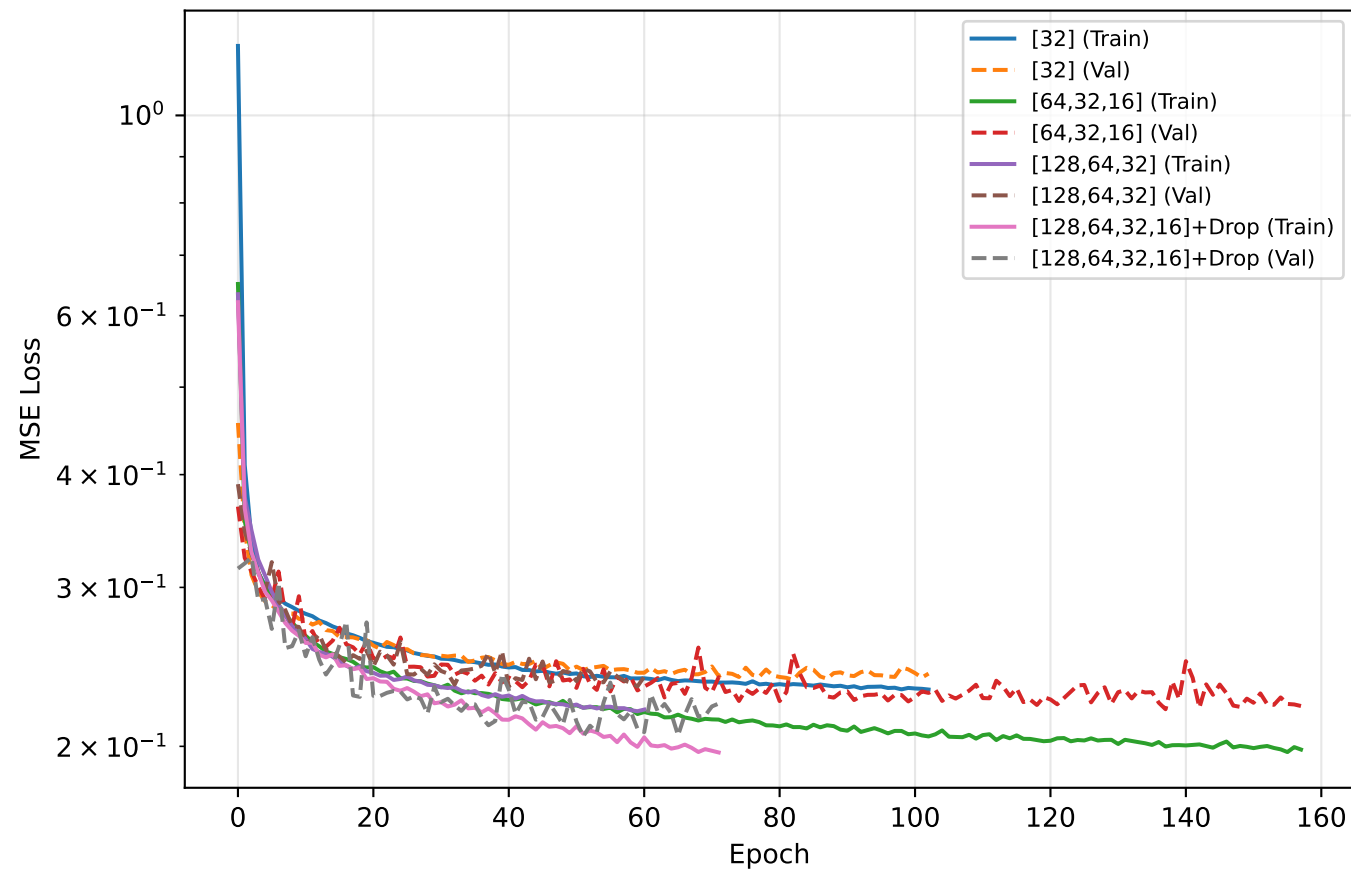
Lernkurven: Loss
