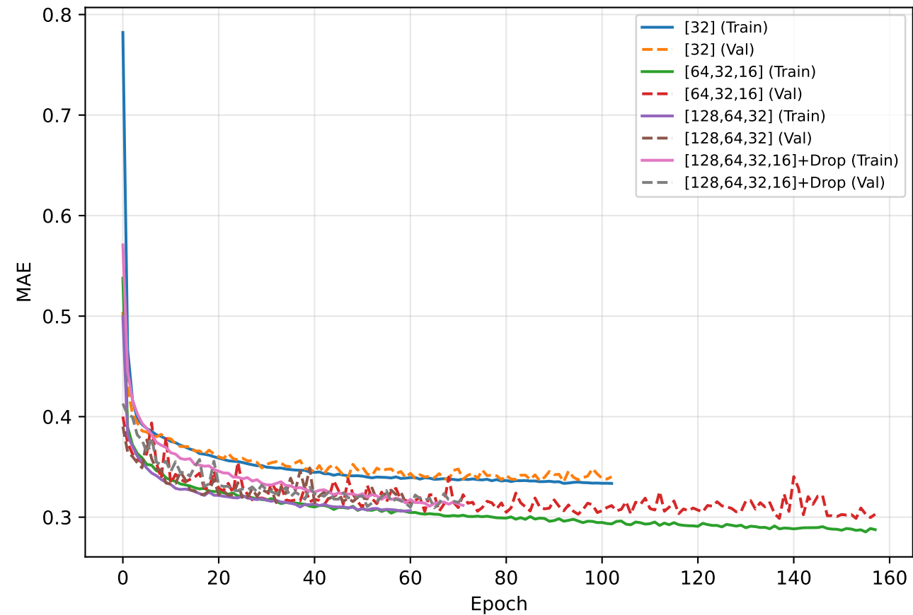
Lernkurven: MAE
