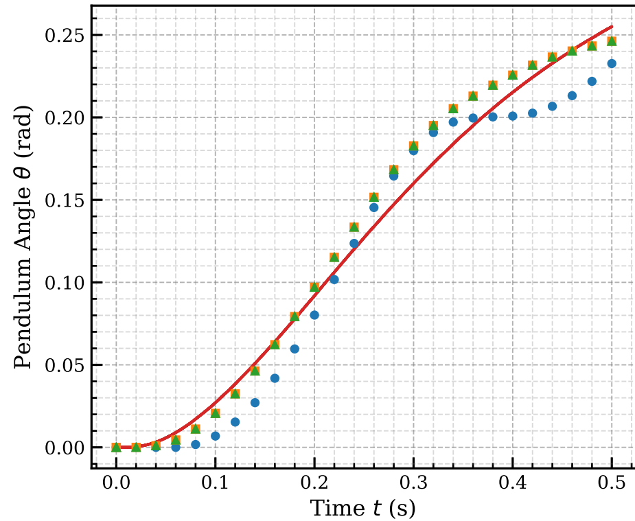
pendulum.q - dt = 0.020 s
