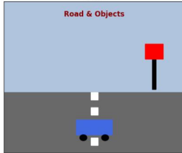
Reflectance r(x,y)
