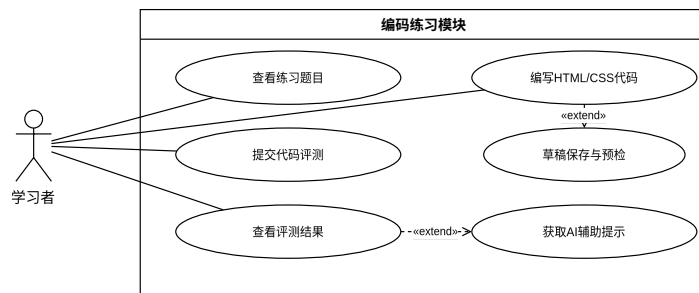
图 3-3 编码练习模块用例图
