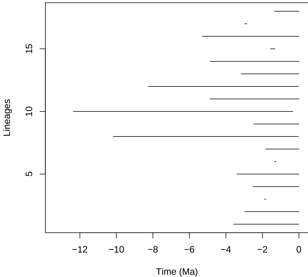
Canis_pbdb_data_1_Grj_mcmc
