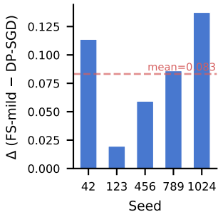
Worst-group F1
