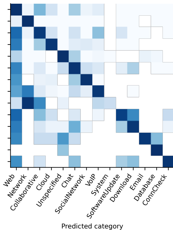
XGBoost / MatchedFlowStats
