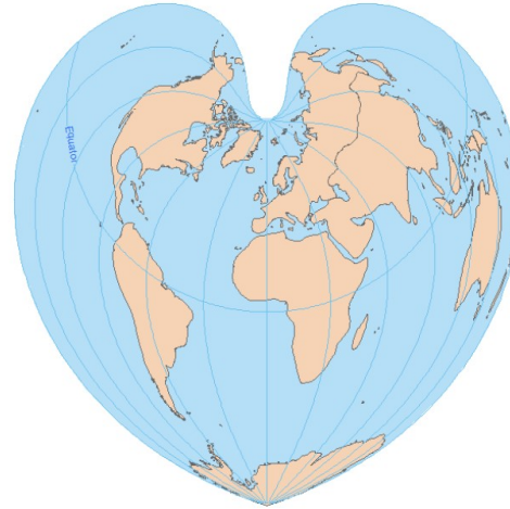
5. Bonne
