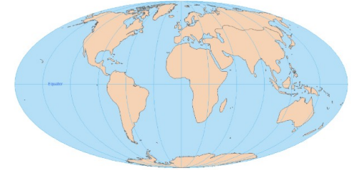
3. Mollweide
