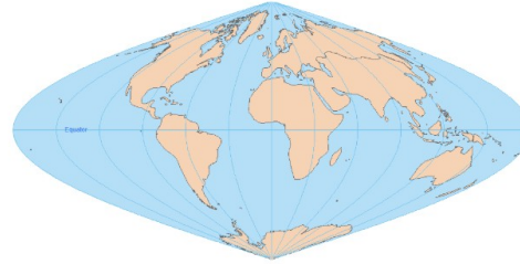
2. Sinusoidal
