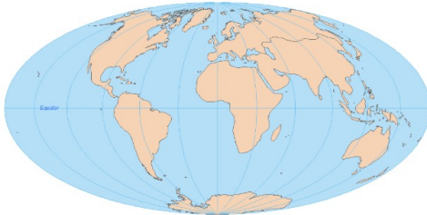
4. Hammer Aitoff
